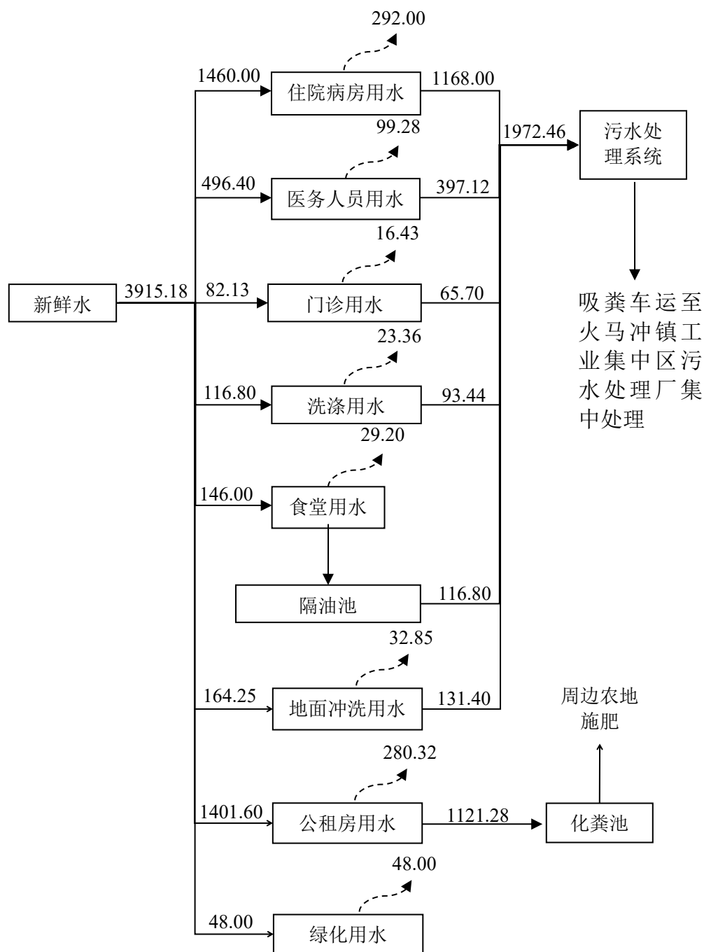
图 2.8-1 项目水平衡图单位: \text{m}^3/\text{a}
