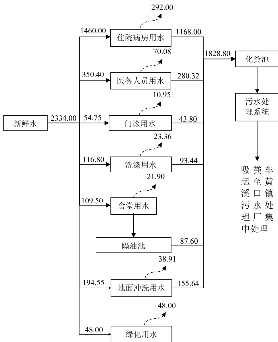
图 2.8-1 项目水平衡图单位：m³/a
