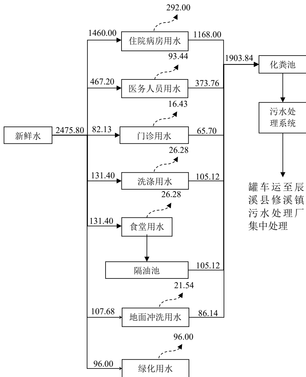
图 2.8-1 项目水平衡图单位: \text{m}^3/\text{a}
